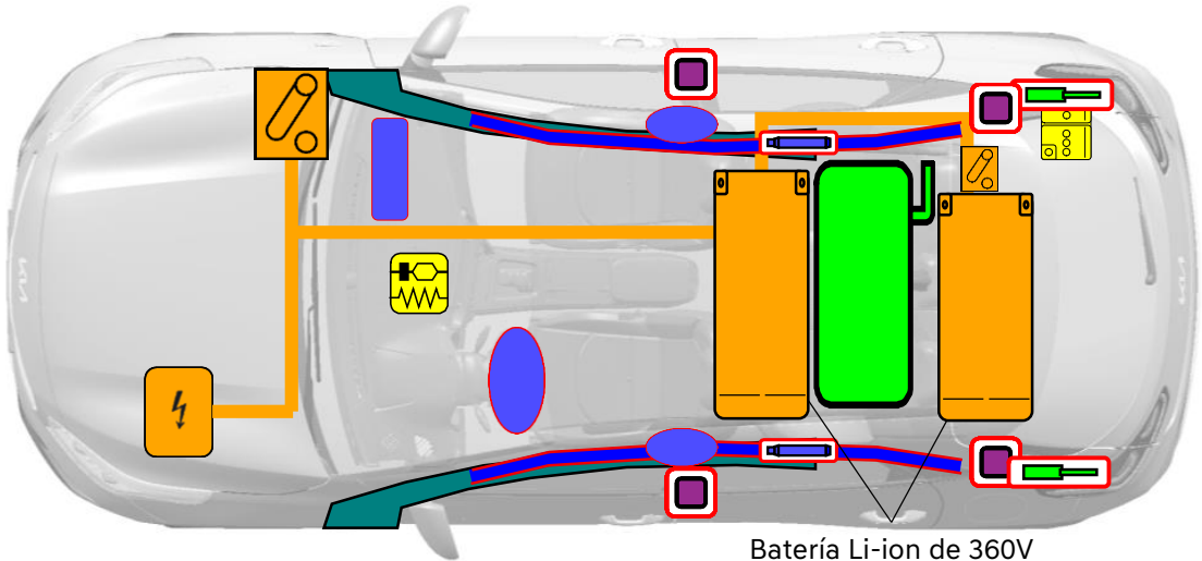
Batería Li-ion de 360V
